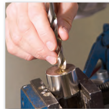
Borrning – Borrskyddet av lås, låscylindrar och beslag provas i maskin.
